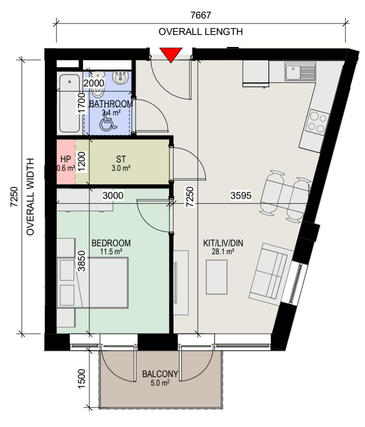
5 Apartment Type 1E 1 : 100
